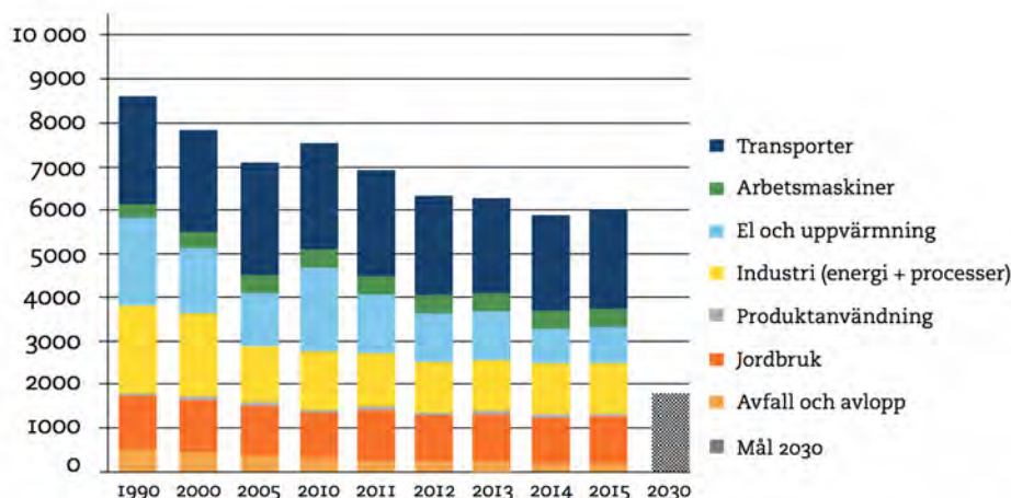
Figur 4 Totala utsläpp av växthusgaser i Skåne per sektor för perioden 1990-2015 och regionalt mål till år 2030 (kton CO 2 ekv). Källa: SMED
